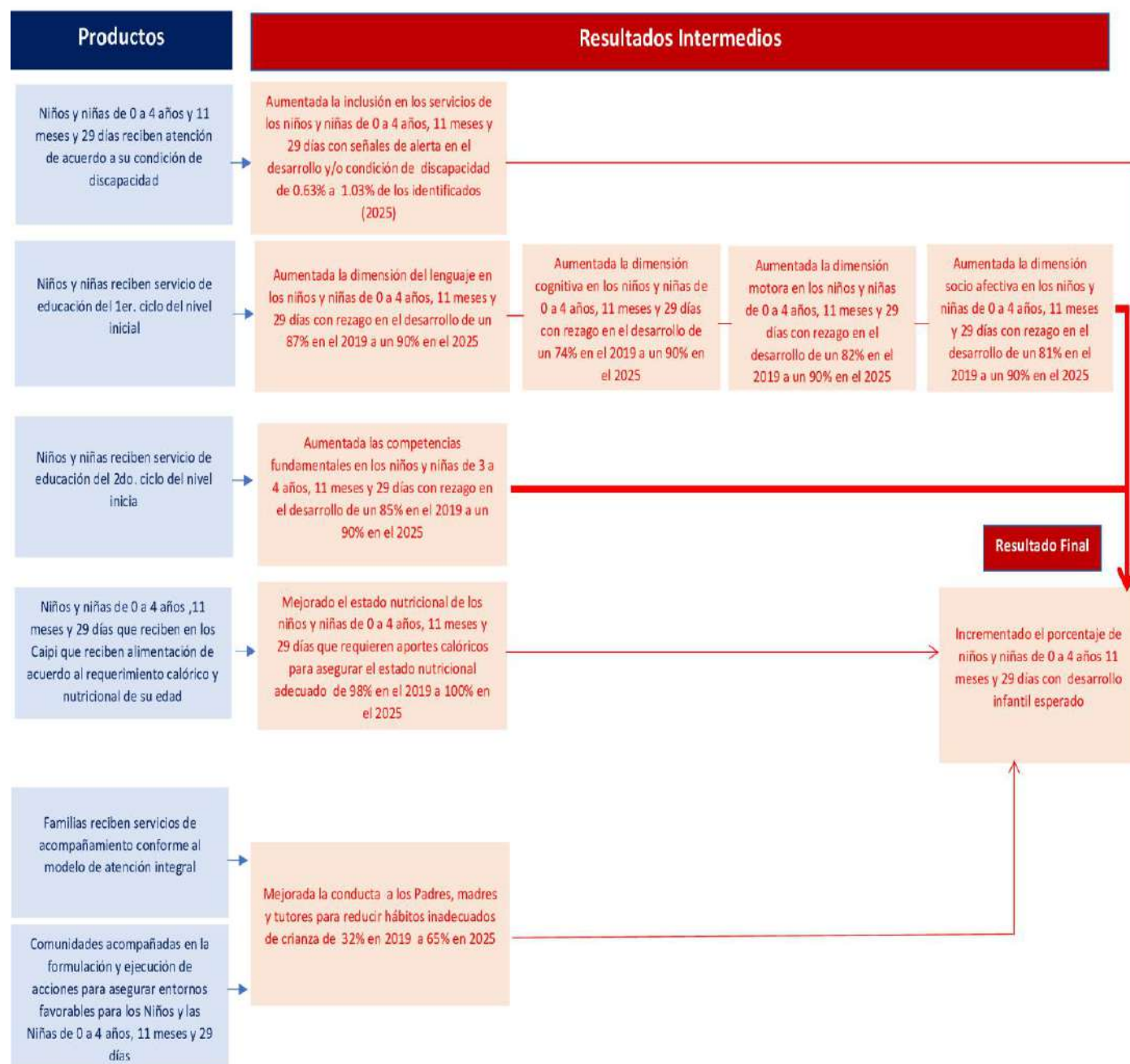
Gráfico 1. Modelo Lógico
