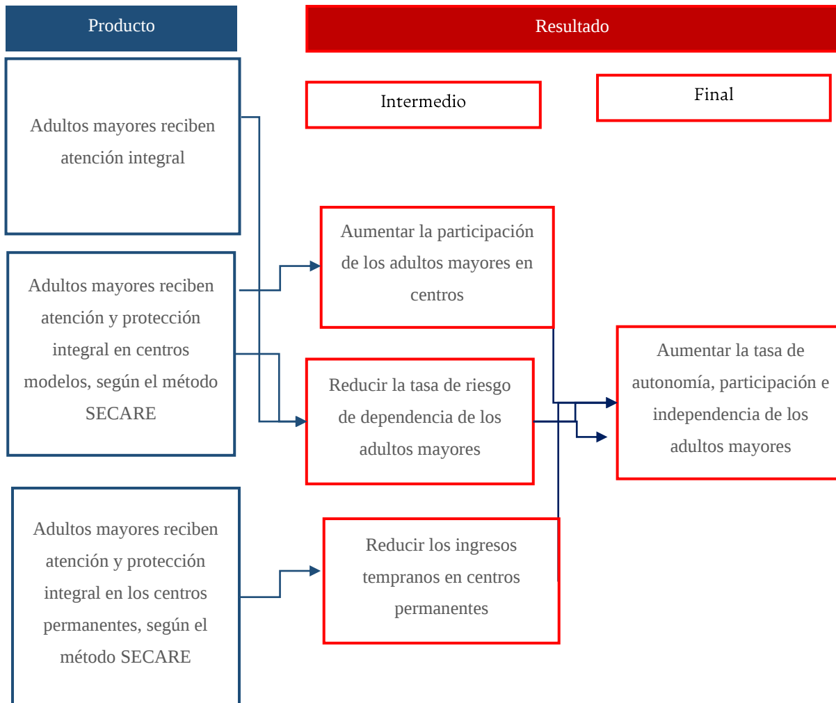
Gráfico 3. Modelo Lógico
