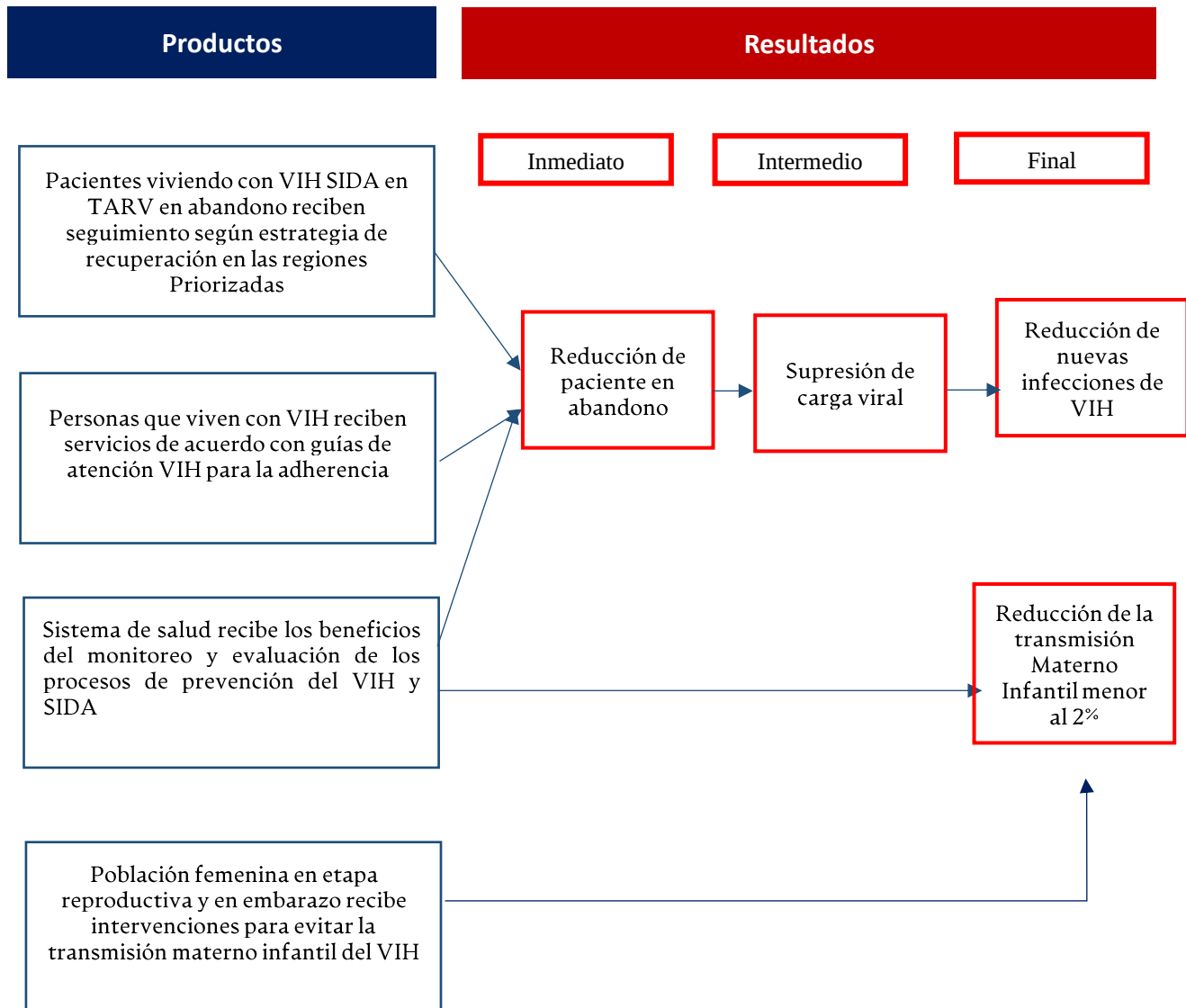
Gráfico 5. Modelo lógico
